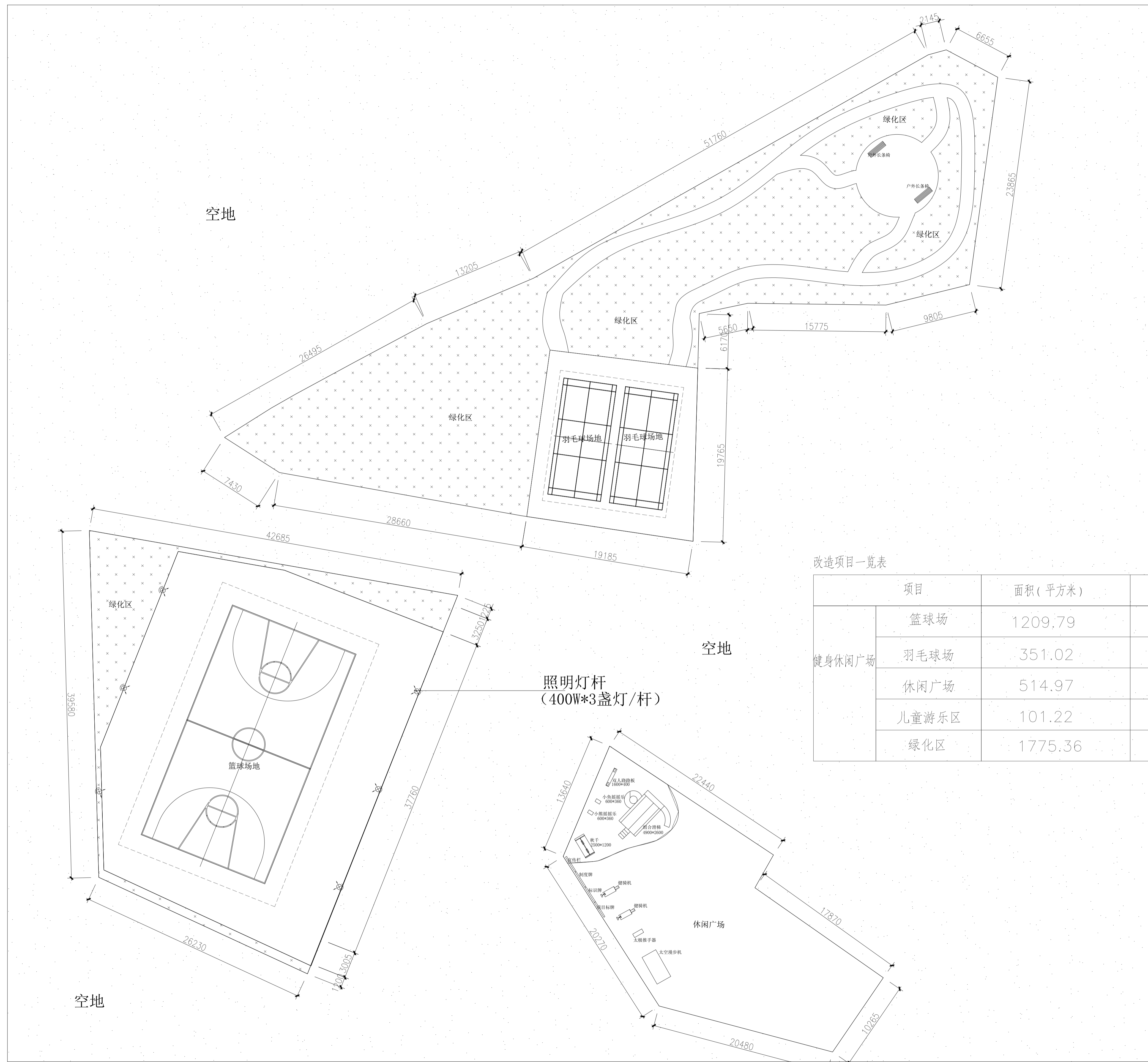
健身休闲广场平面图 1:1000
